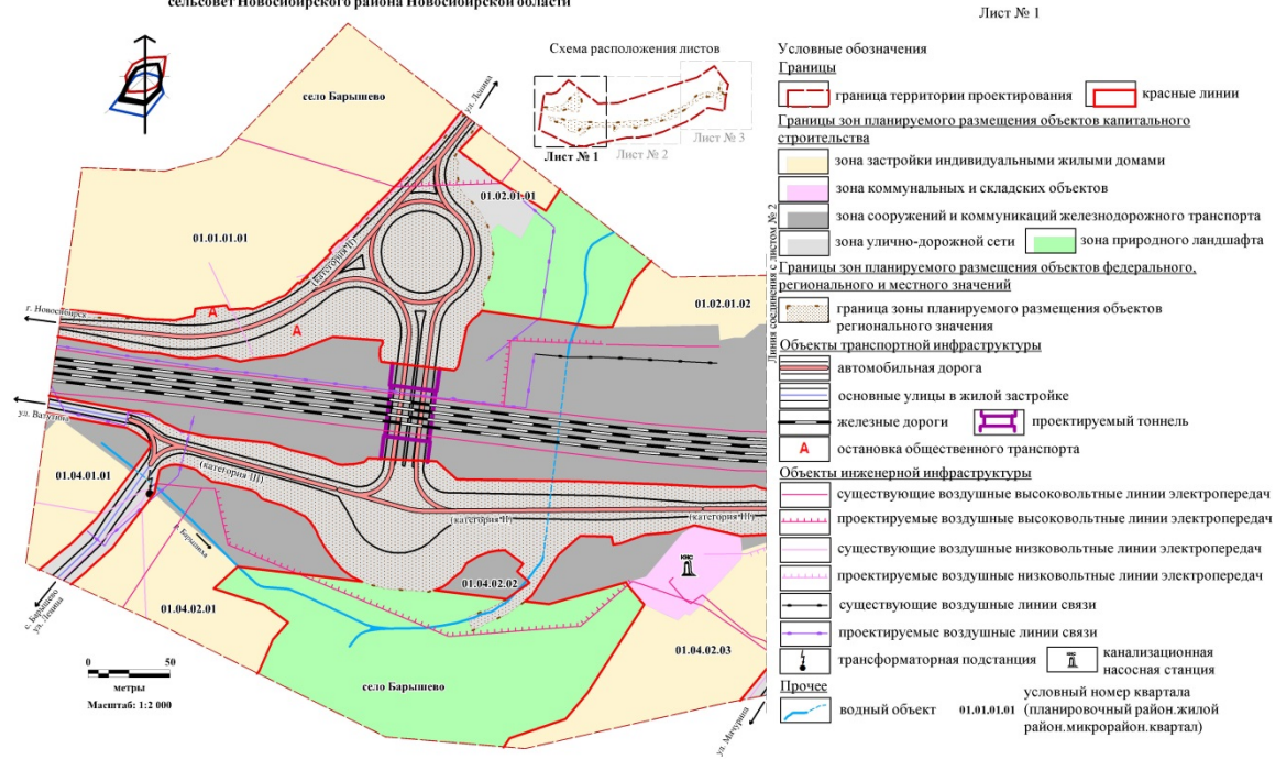
Чертеж планировки территории для размещения объекта регионального значения автомобильной дороги «Барышево – Орловка – Кольцово» с автодорожным тоннелем под железной дорогой в границах муниципальных образований рабочий поселок Кольцово и Барышевский сельсовет Новосибирского района Новосибирской области
